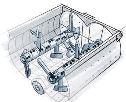
Doppelwellenmischer
